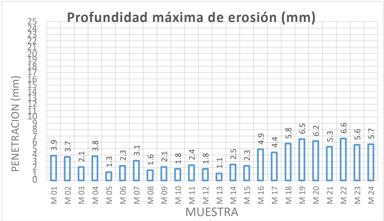
Ilustración 44 Diagrama de barras resultados profundidad de erosión por erosión para granulometría G9
