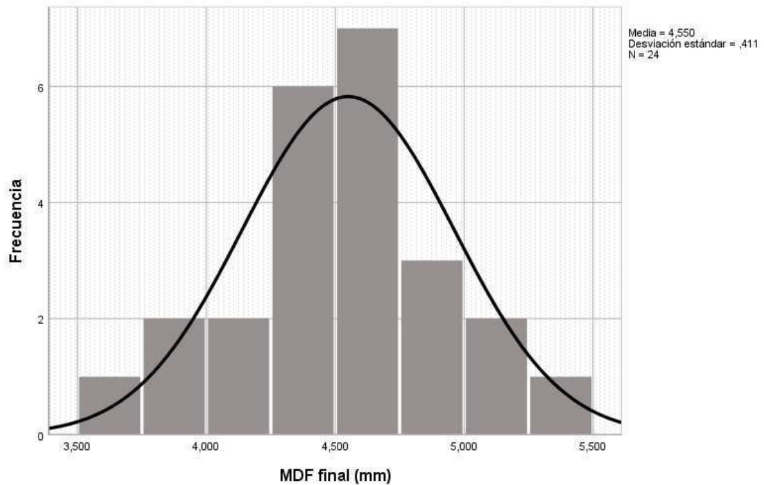
Ilustración 63 Histograma - MDF final (mm)
