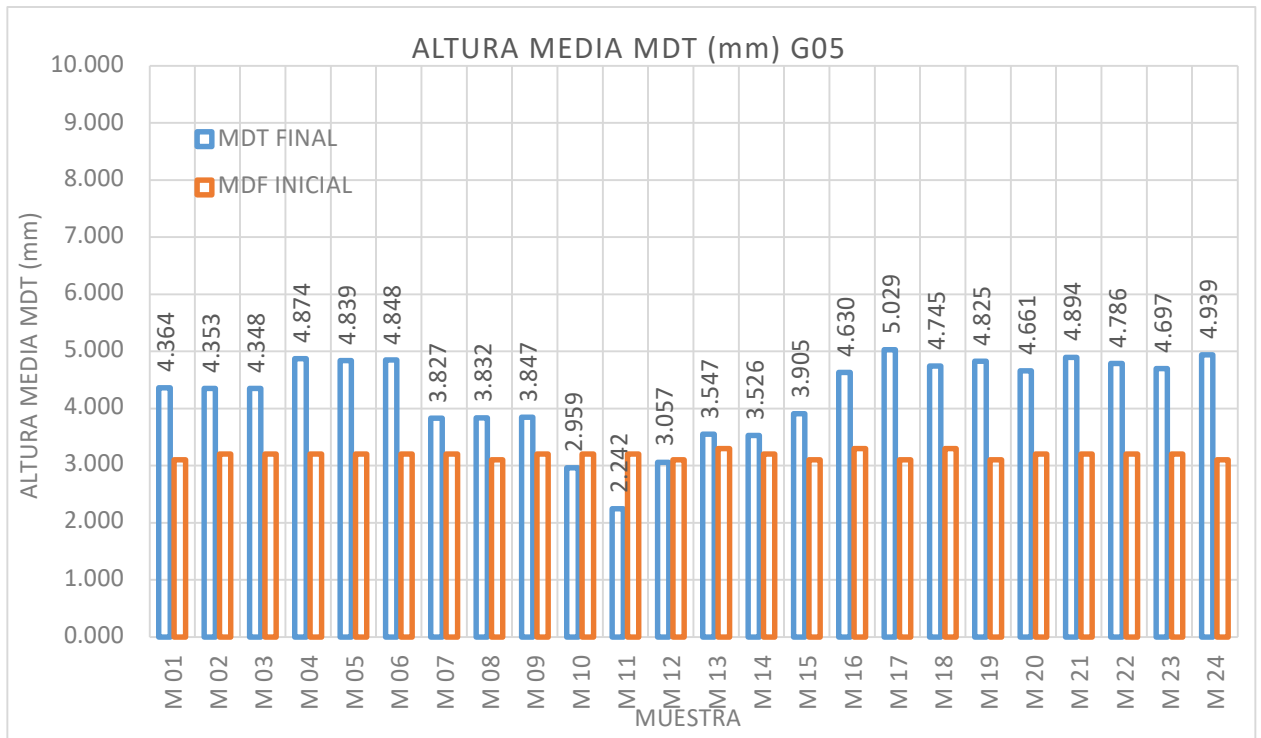
Ilustración 46 Diagrama de barras resultados del MDT inicial y MDT final del ensayo de circulo de arena para granulometría G5
