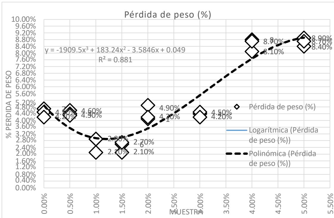
Ilustración 35 Gráfica de tendencia resultados pérdida de peso por erosión acelerada para granulometría G7
