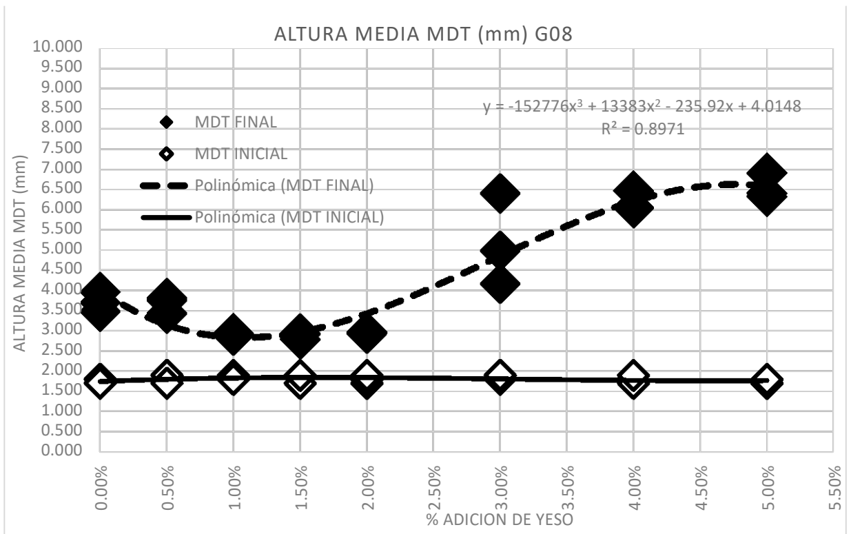
Ilustración 53 Gráfica de tendencia de resultados del MDT inicial y MDT final del ensayo de círculo de arena para granulometría G8
