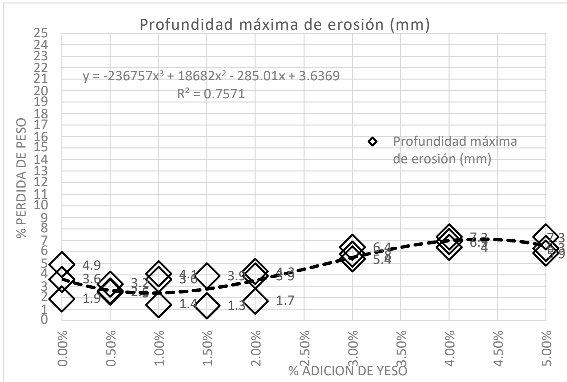
Ilustración 29 Gráfica de tendencia resultados profundidad de erosión por erosión para granulometría G5
