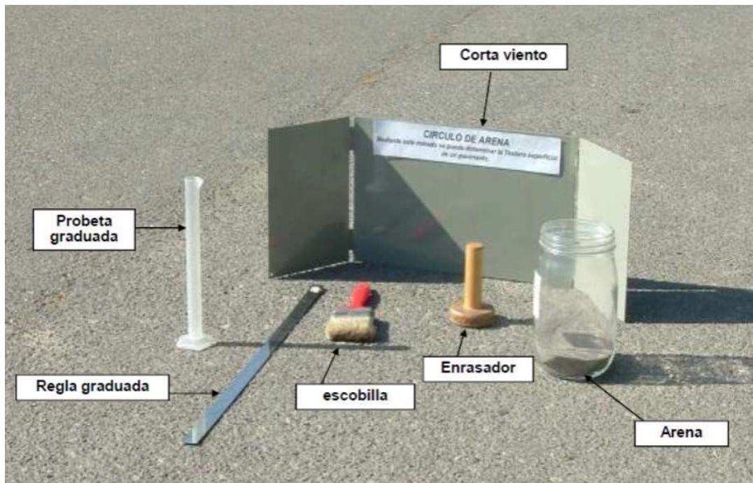
Ilustración 5 Lista de equipos para ensayo de círculo de arena
