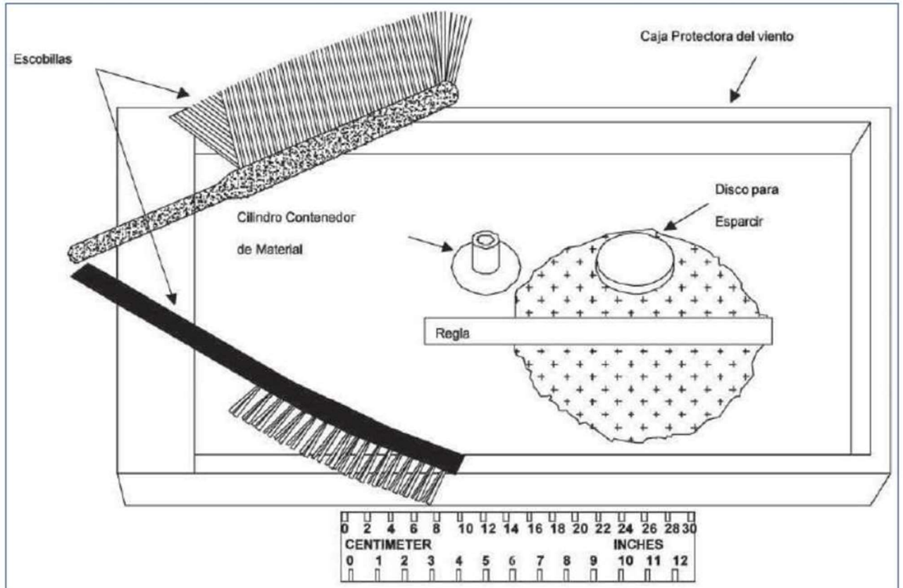
Ilustración 11 APARATO PARA MEDIR PROFUNDIDAD DE MACROTEXTURA DE LA SUPERFICIE DEL PAVIMENTO
