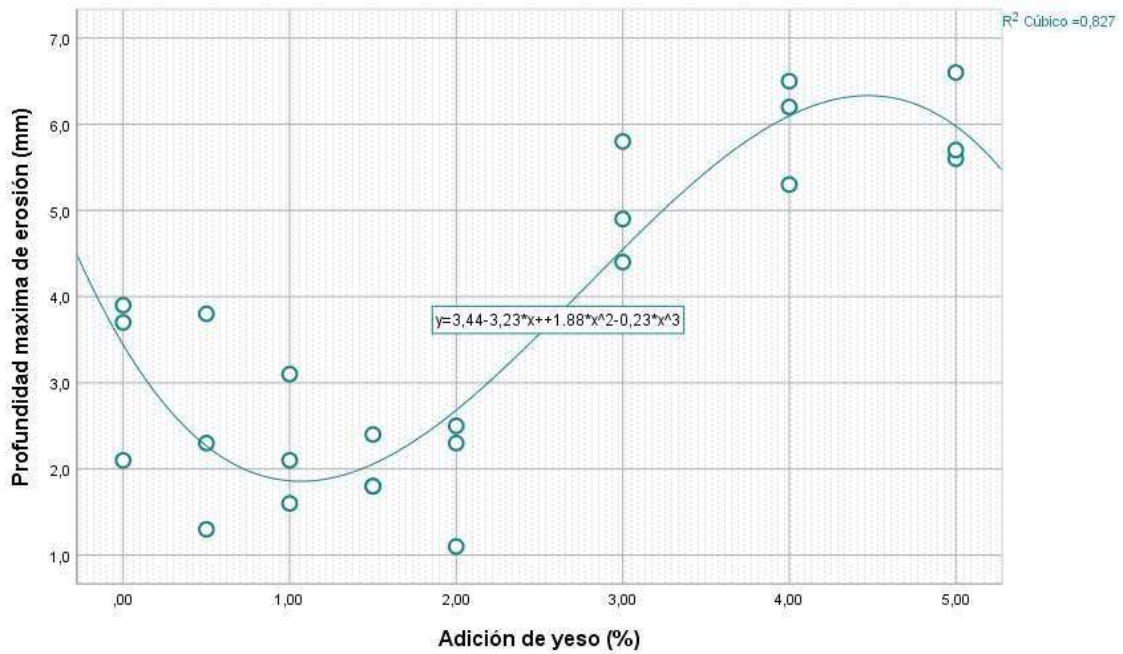
Ilustración 62 Diagrama de dispersión de puntos - Profundidad máxima de erosión (mm) Fuente: Elaboración propia
