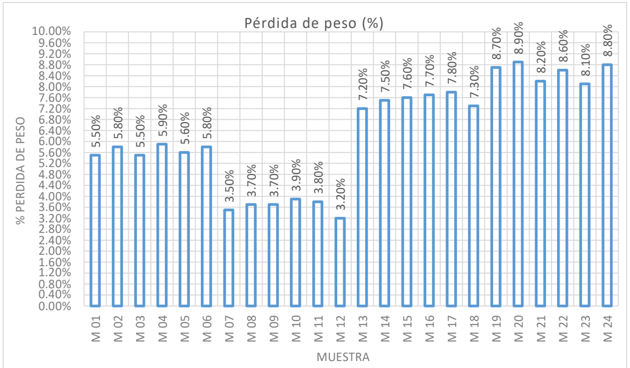
Ilustración 42 Diagrama de barras resultados pérdida de peso por erosión acelerada para granulometría G9
