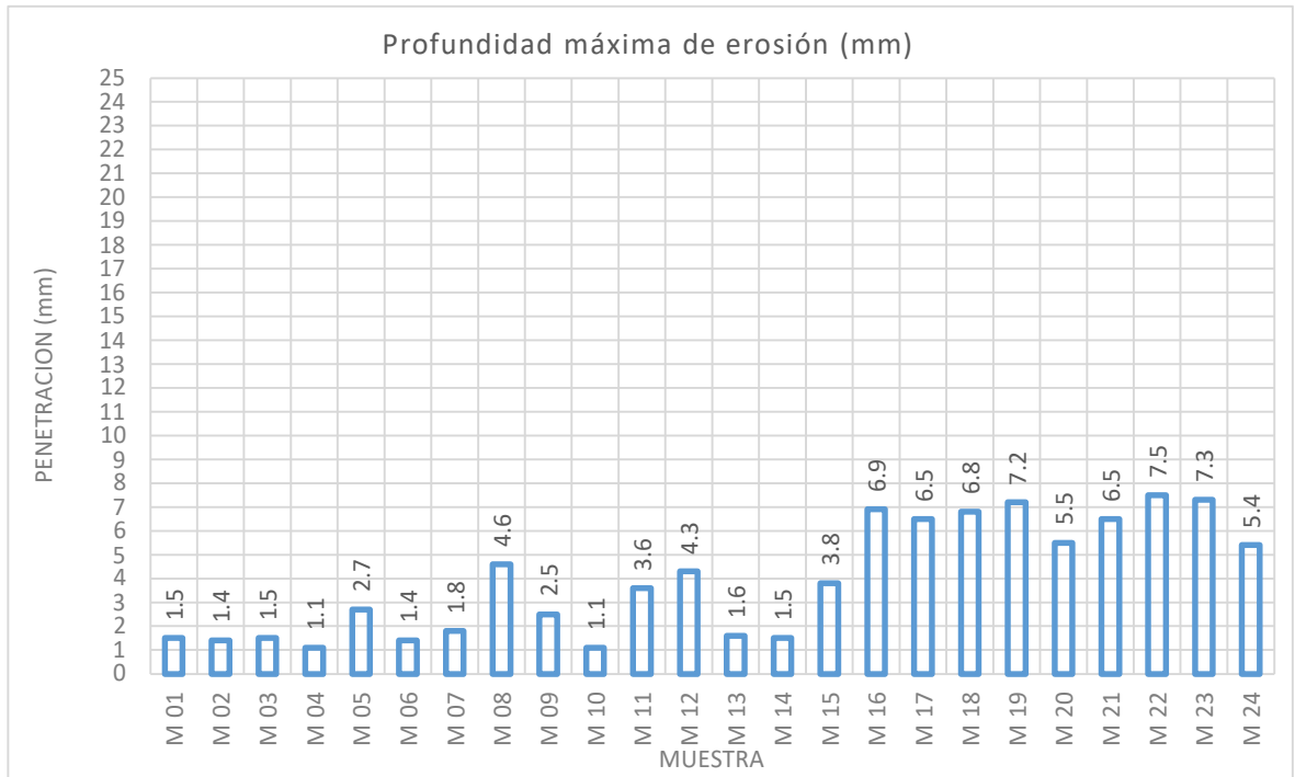
Ilustración 32 Diagrama de barras resultados profundidad de erosión por erosión para granulometría G6
