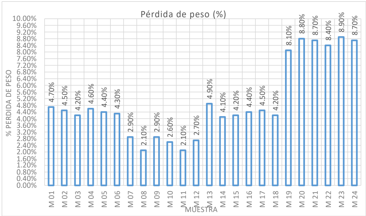
Ilustración 34 Diagrama de barras resultados pérdida de peso por erosión acelerada para granulometría G7
