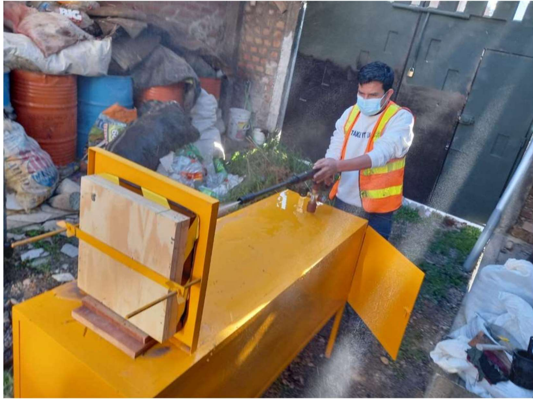
Ilustración 80 Ensayo de Daño por Erosión
