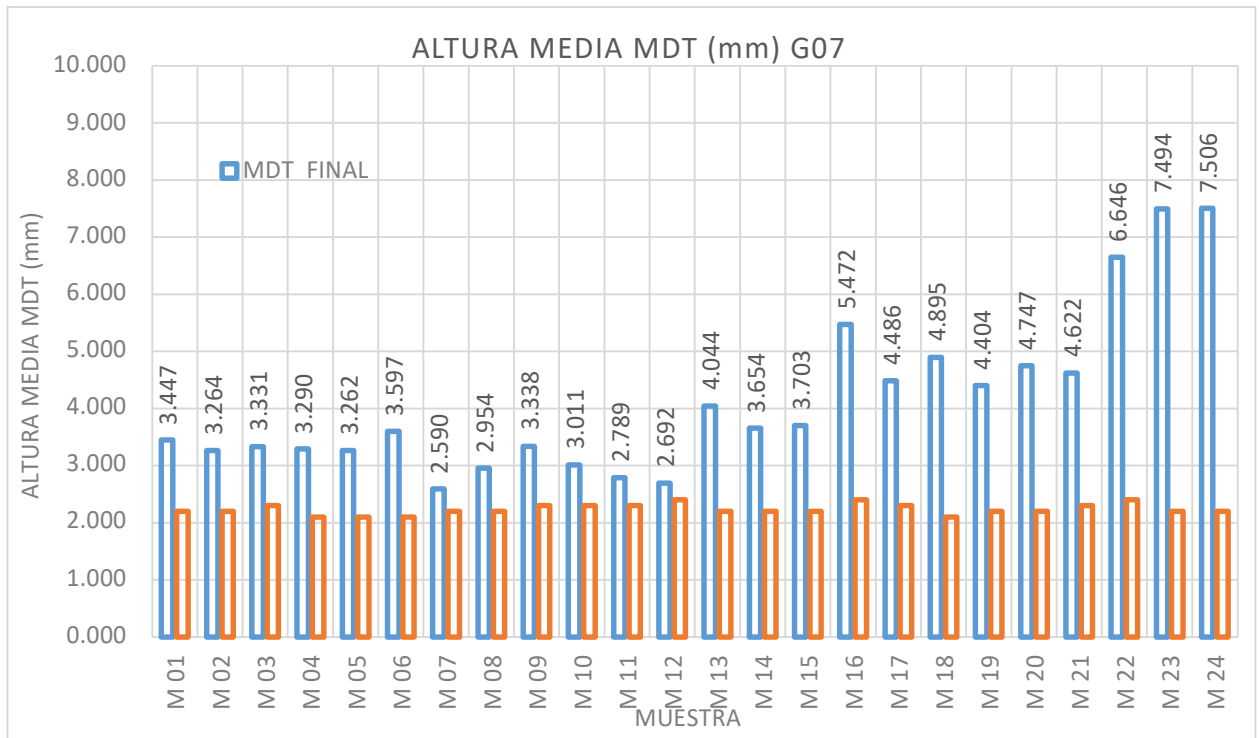
Ilustración 50 Diagrama de barras resultados del MDT inicial y MDT final del ensayo de circulo de arena para granulometría G7
