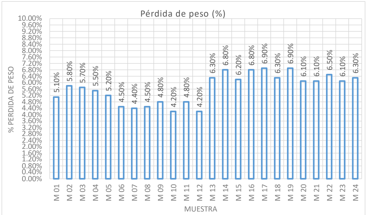
Ilustración 38 Diagrama de barras resultados pérdida de peso por erosión acelerada para granulometría G8
