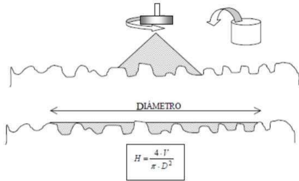
Ilustración 10 Esquema del esparcido de la arena en el pavimento.
