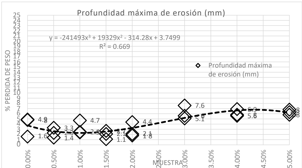
Ilustración 41 Gráfica de tendencia resultados profundidad de erosión por erosión para granulometría G8
