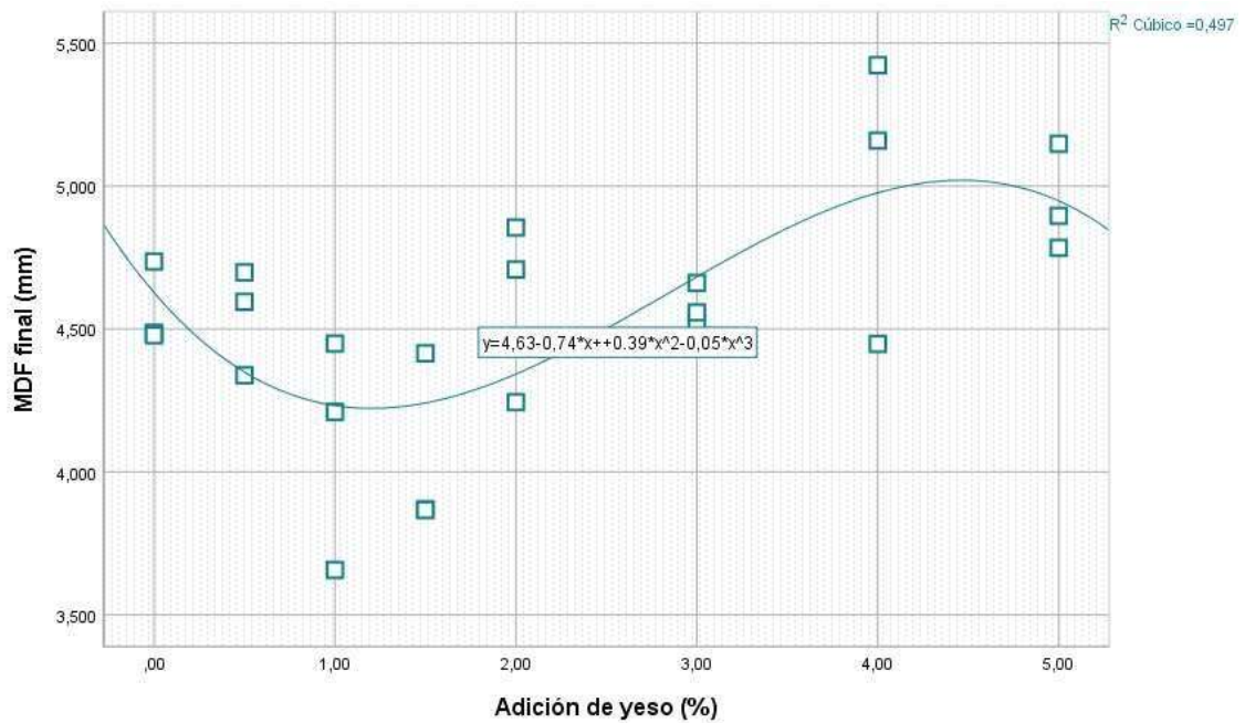
Ilustración 64 Diagrama de dispersión de puntos - MDF final (mm)
