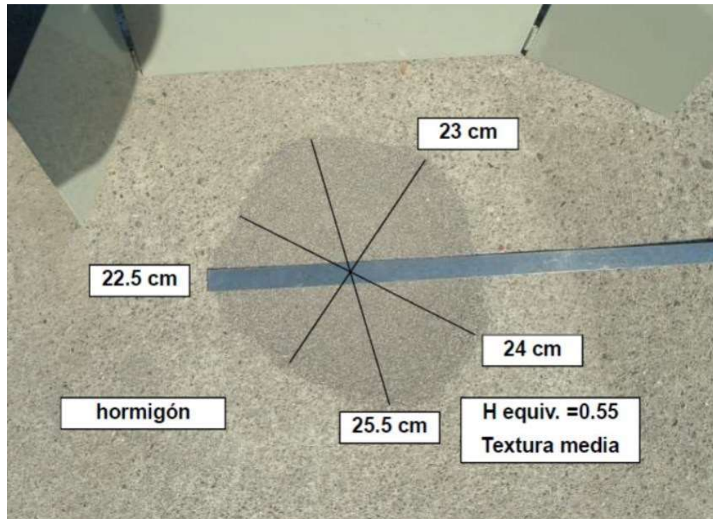
Ilustración 9 Múltiples mediciones del diámetro del círculo de arena formado
