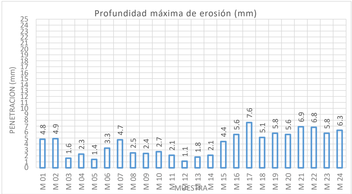
Ilustración 40 Diagrama de barras resultados profundidad de erosión por erosión para granulometría G8
