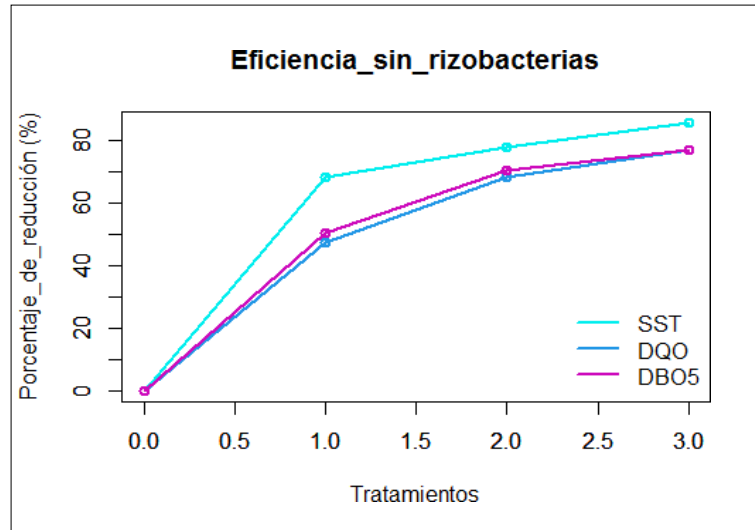
Figura 8. Eficiencia del tratamiento de AR con HA.
