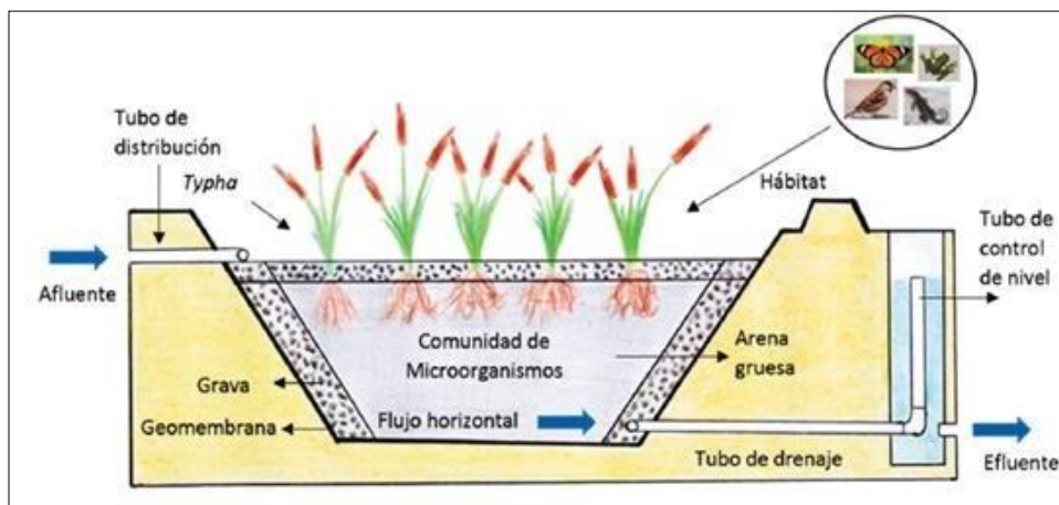
Figura 1. Humedal de flujo sub superficial horizontal (FSSH).
