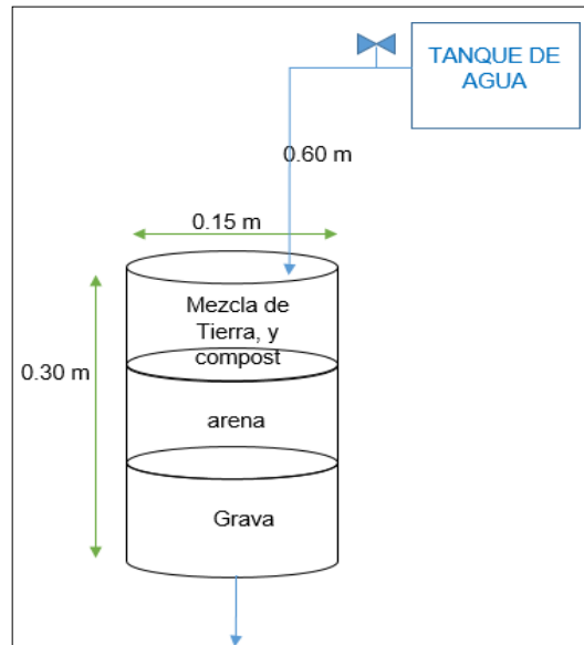
Figura 7. Diseño del humedal artificial.
