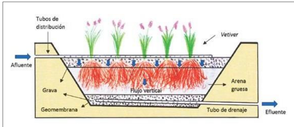
Figura 2. Humedal de flujo sub superficial vertical (FSSV).
