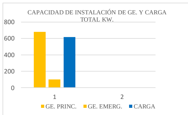
Fig.9 Capacidad de potencia instalada y carga instalada
