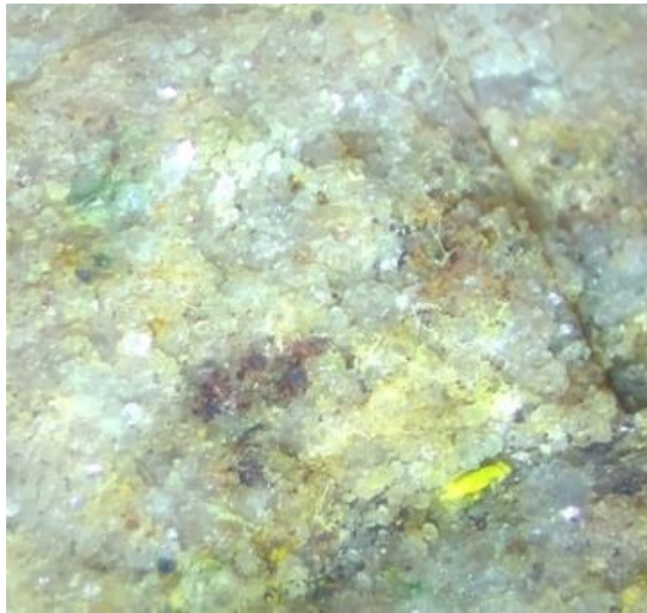
Imagen 5: Muestra microscópica de calcita
