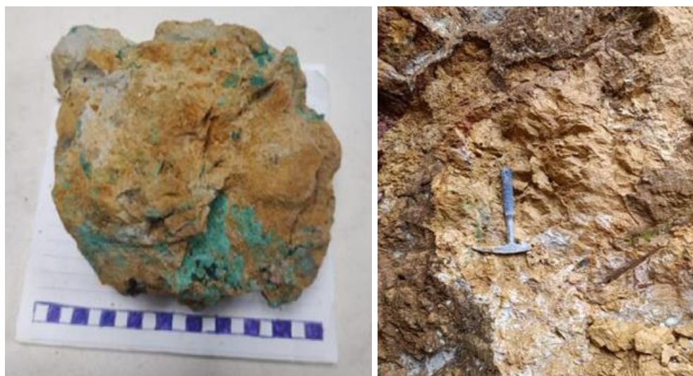
Imagen 8. Foto macroscópica de limonita
