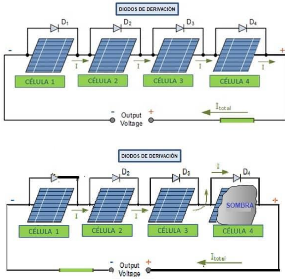
Figura 9. La tecnología FV. Tomada de: Future of Solar Energy , por International Renewable Energy Agency (IRENA), 2020.
