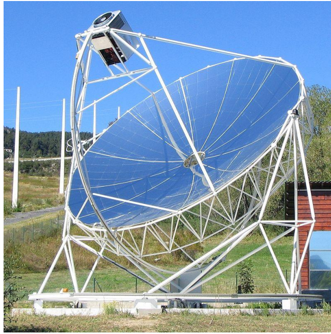
Figura 3. Platos Stirling. Tomada de: Platos Stirling y su uso en energía solar, por Renewable Energy World, 2019.
