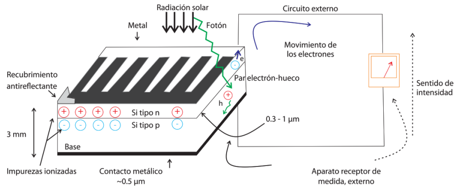
Figura 7. Células fotovoltaicas. Tomada de: Physics of Solar Cells , por Chiang, 2016.
