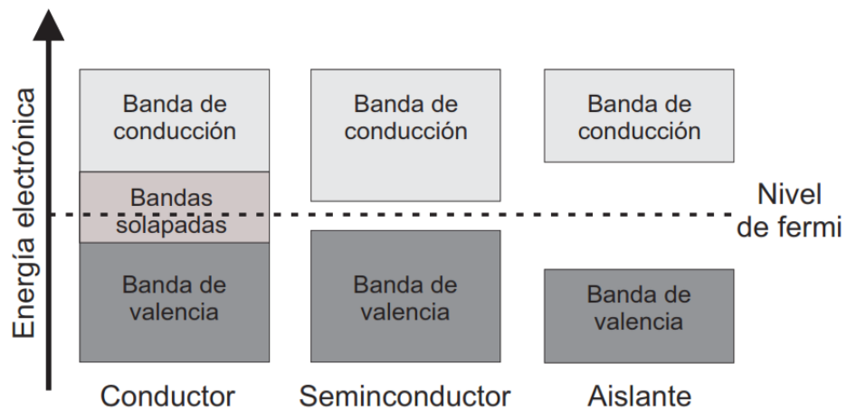
Figura 6. Bandas de energía. Tomada de: Physics of Solar Cells, por Chiang, 2016.
