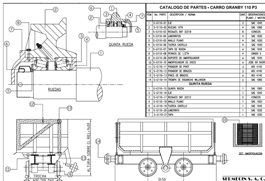
Figura 14: Partes del carro minero Gramby Fuente: Tomada de GMI
