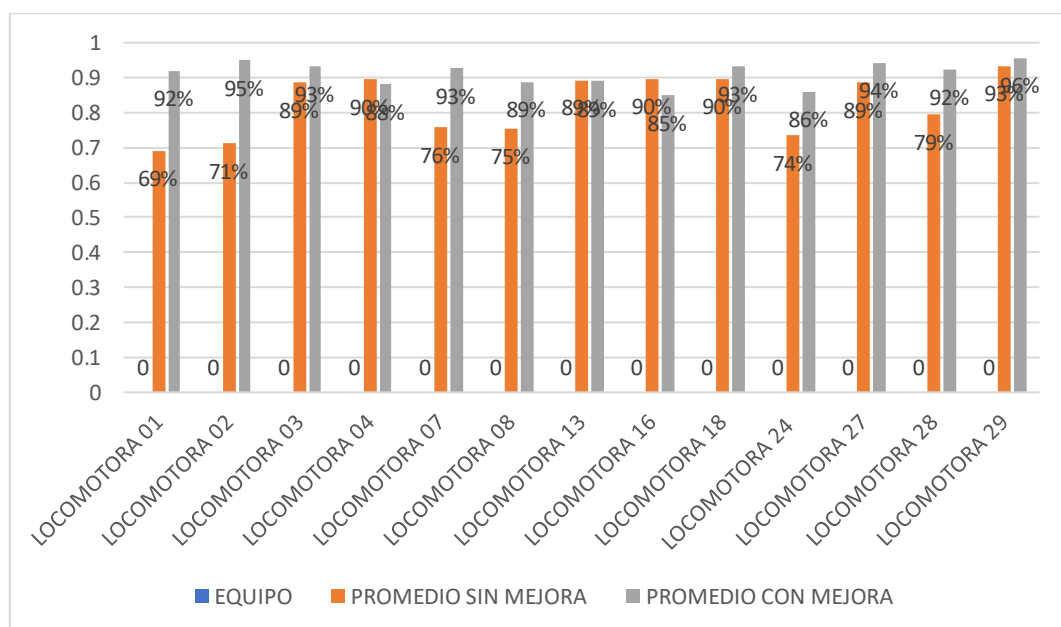
Figura 45. Comparativa de promedios registrados de disponibilidad
