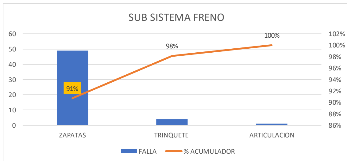
Figura 22. Diagrama por fallas de subsistemas – freno
