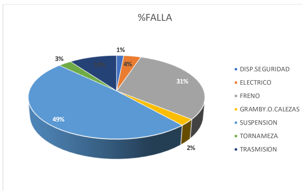
Figura 9: Falla por sistemas
