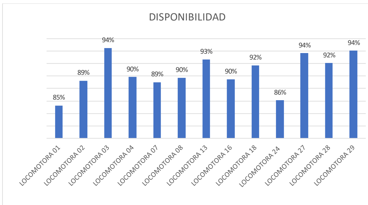
Figura 31. Grafica de disponibilidades mejorada
