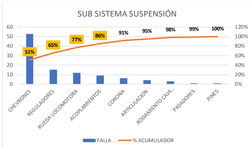
Figura 21. Diagrama por fallas de subsistemas suspensión
