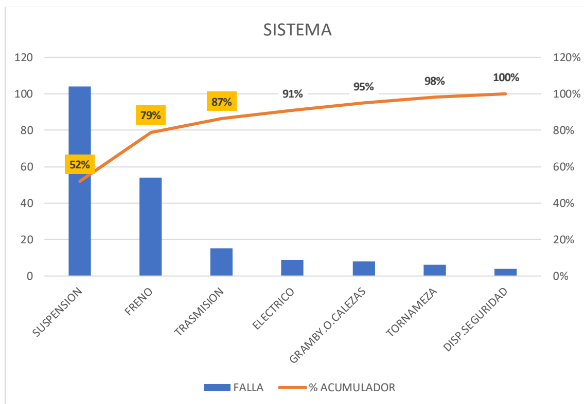
Figura 20. Diagrama por fallas de sistemas
